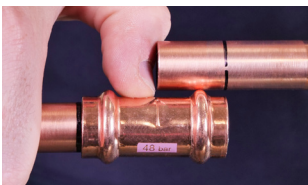
9. Markierung überprüfen
