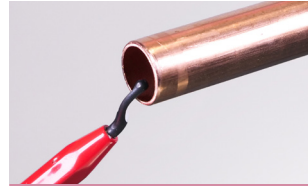
3. Rohr innen und außen entgraten
